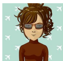
「クッキー」
